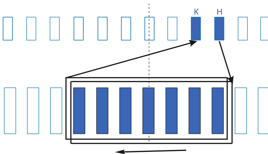
Схема намотки
