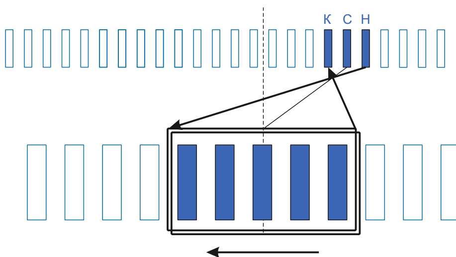
Схема намотки
