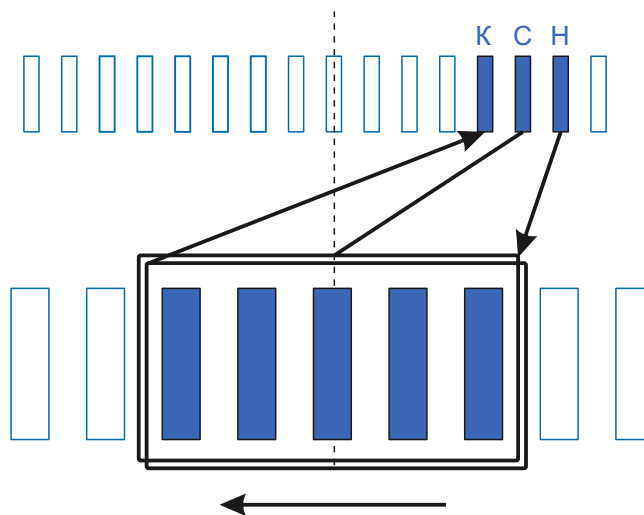
Схема намотки
