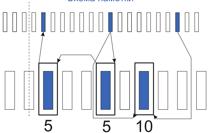
Схема намотки
