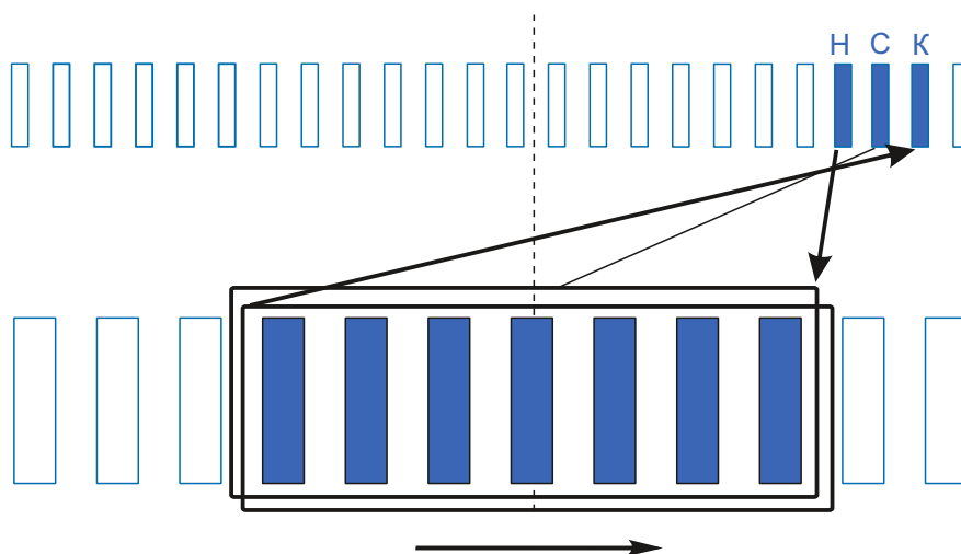
Схема намотки
