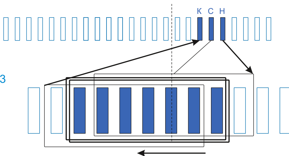
Схема намотки
