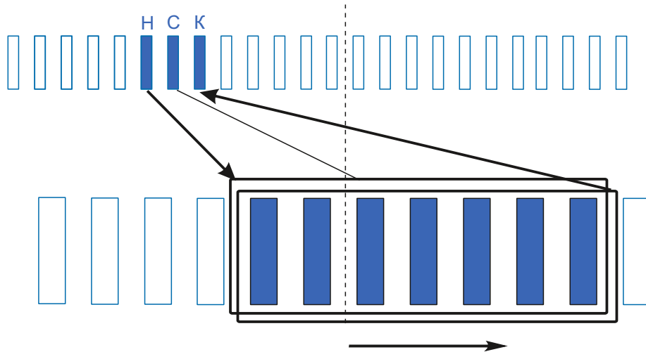
Схема намотки
