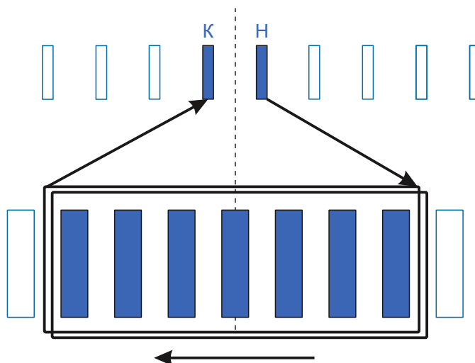
Схема намотки
