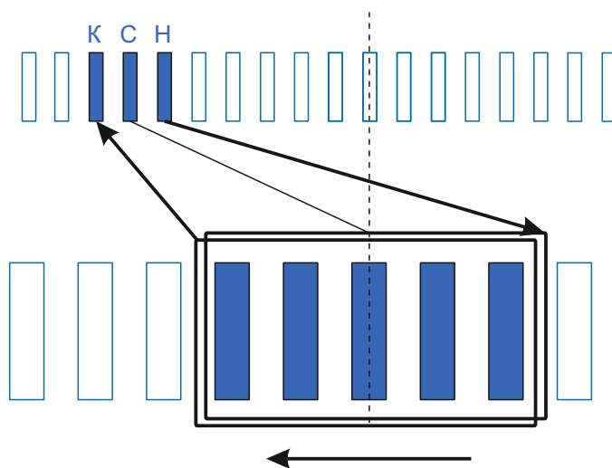
Схема намотки
