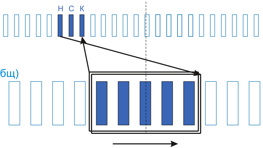
Схема намотки
