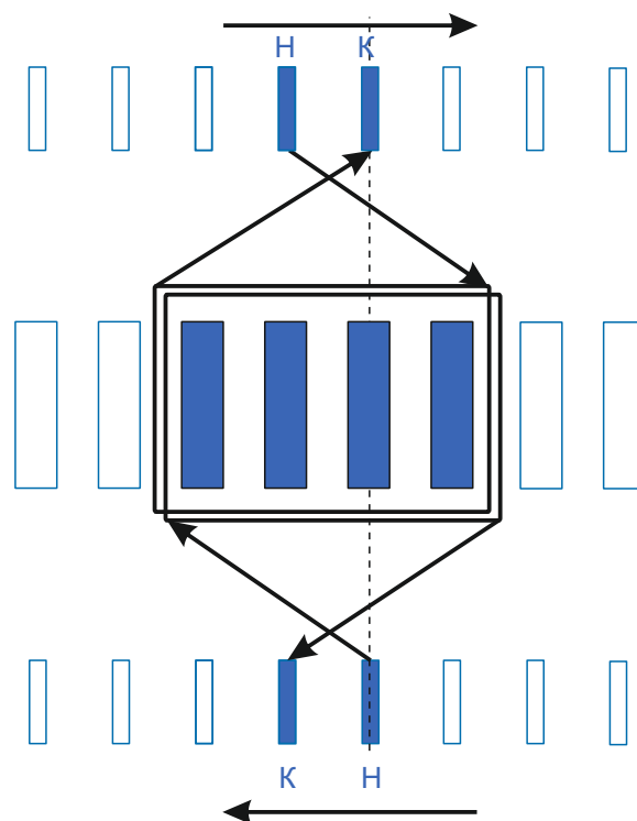
Схема намотки
