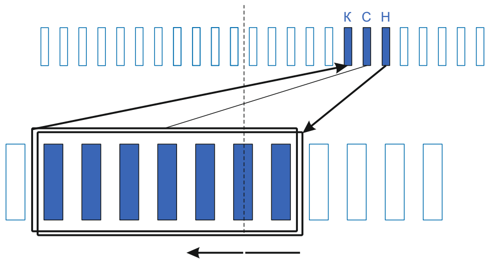
Схема намотки
