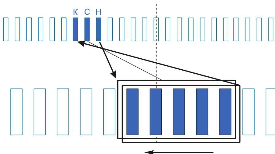
Схема намотки
