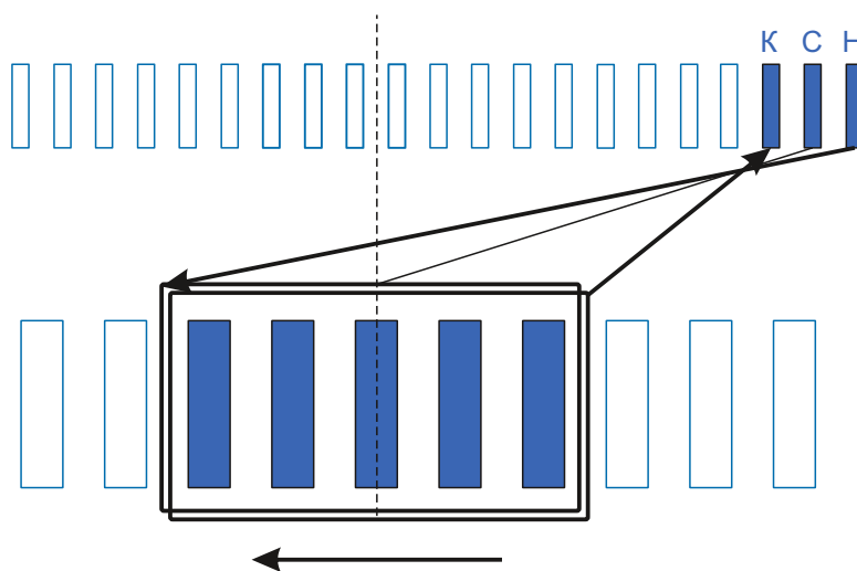
Схема намотки
