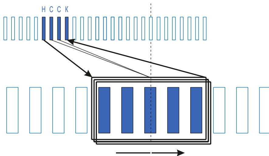
Схема намотки
