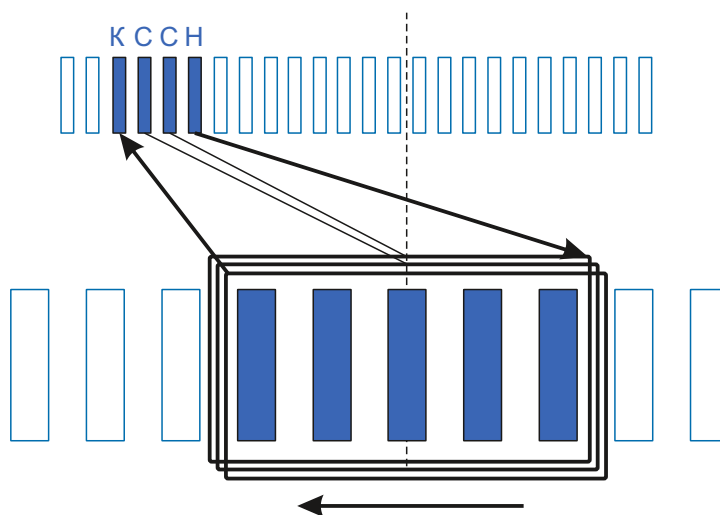
Схема намотки
