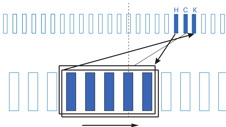
Схема намотки
