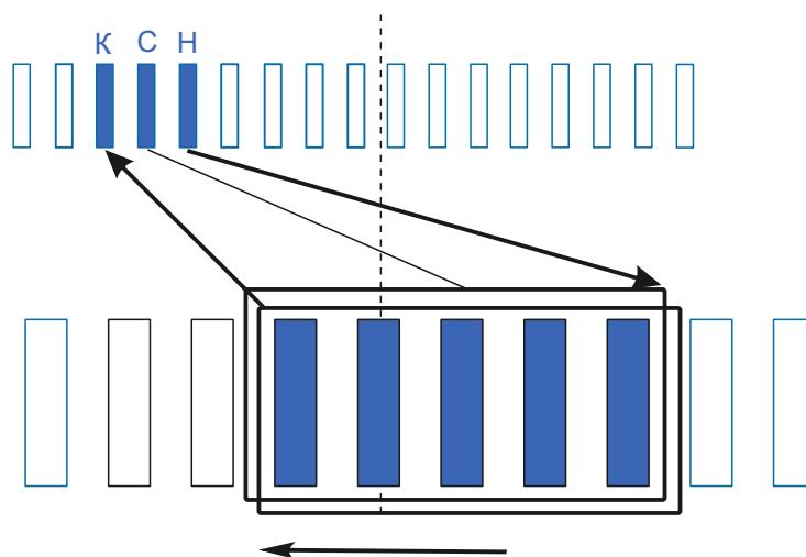
Схема намотки
