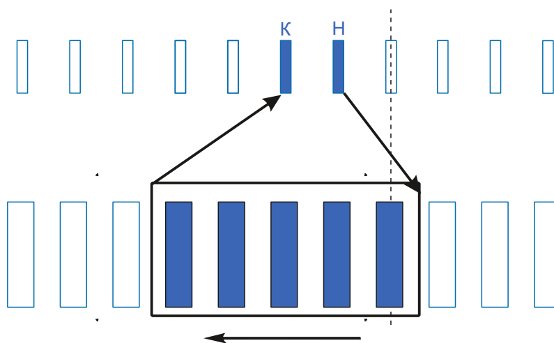
Схема намотки
