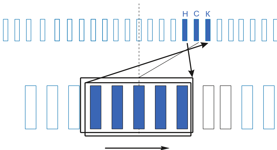
Схема намотки
