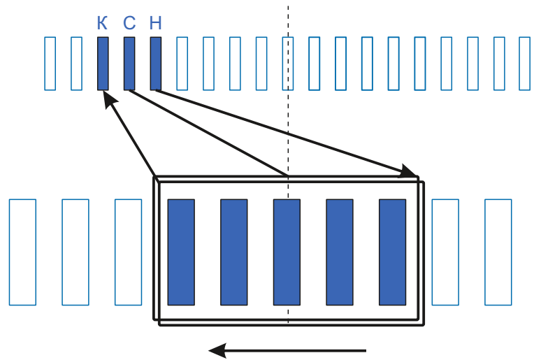
Схема намотки
