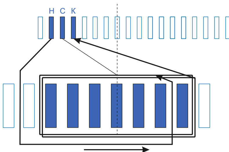
Схема намотки
