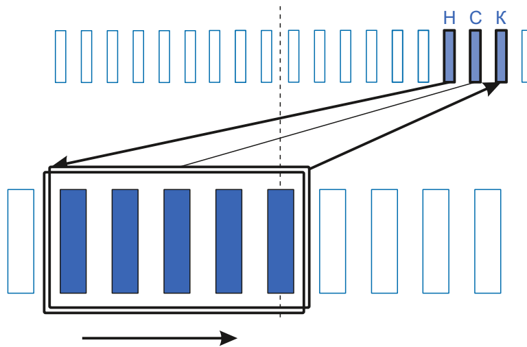
Схема намотки
