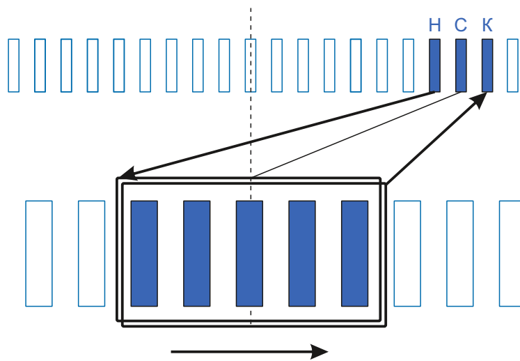
Схема намотки
