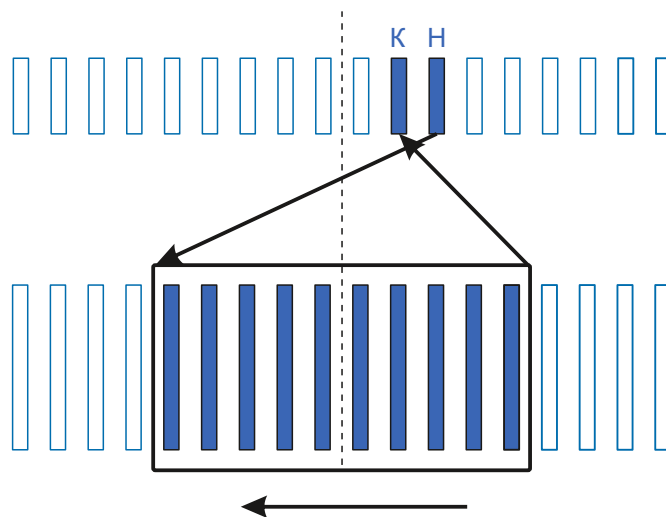
Схема намотки
