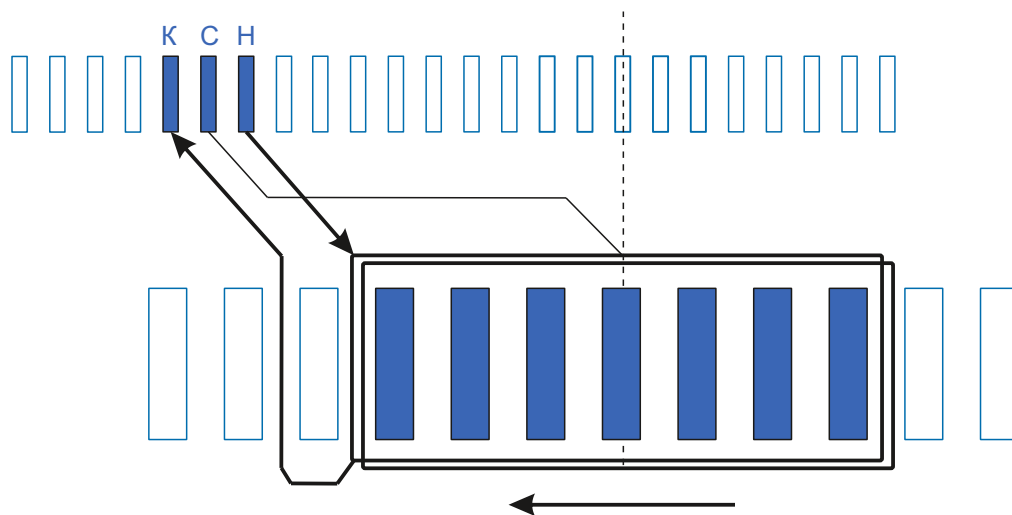
Схема намотки
