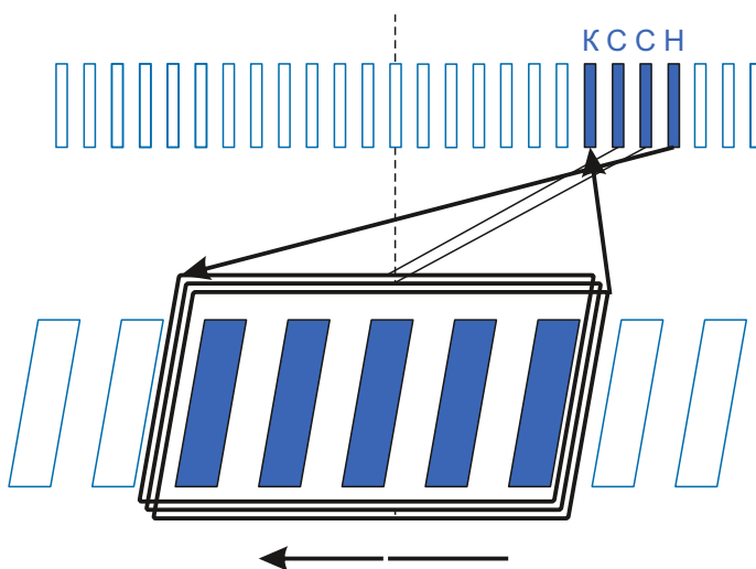
Схема намотки
