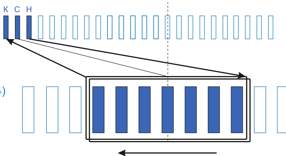
Схема намотки
