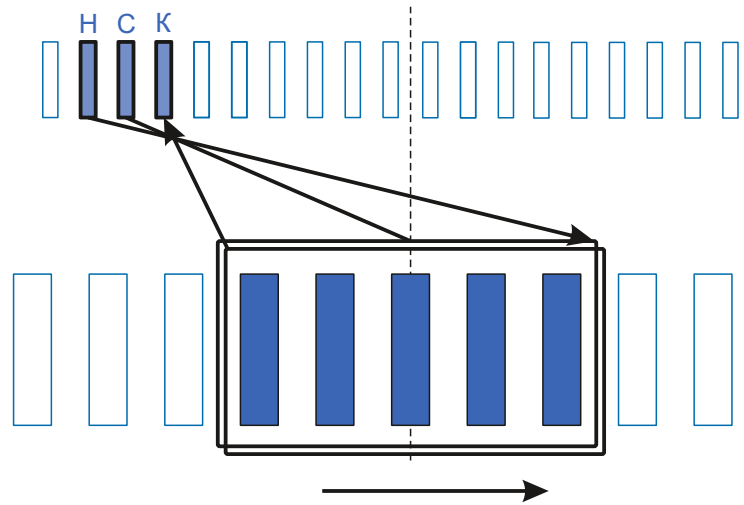
Схема намотки
