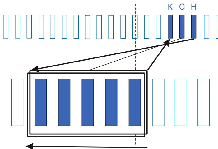
Схема намотки
