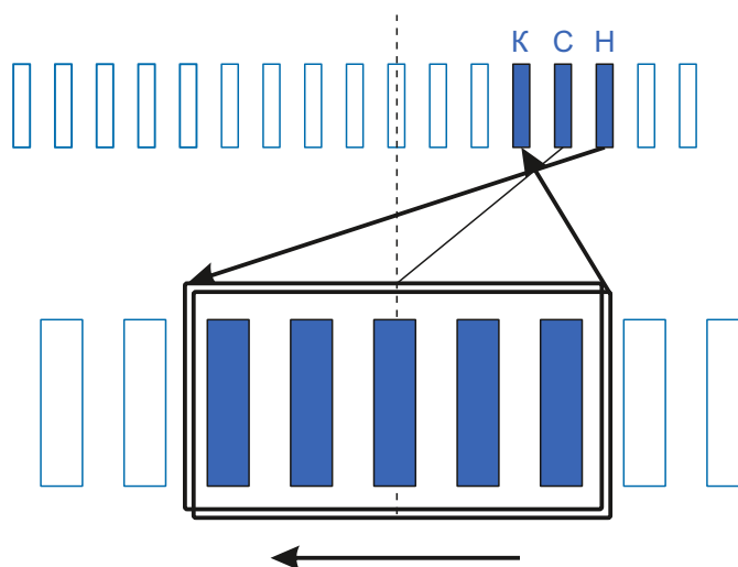
Схема намотки
