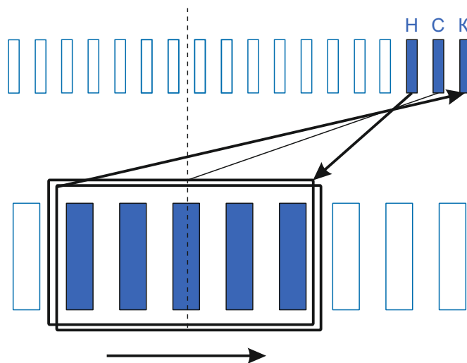
Схема намотки
