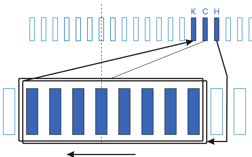
Схема намотки
