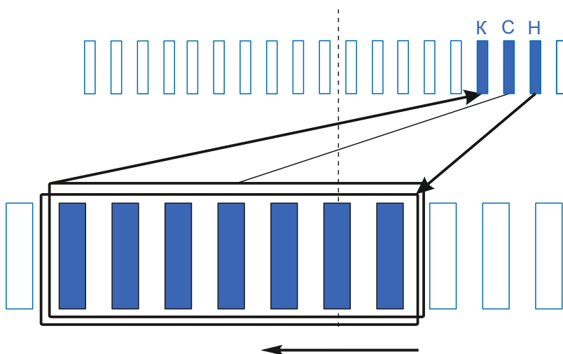
Схема намотки
