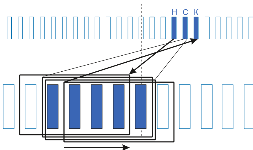
Схема намотки
