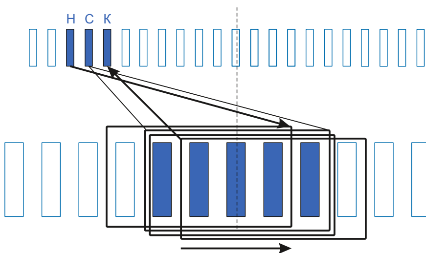
Схема намотки
