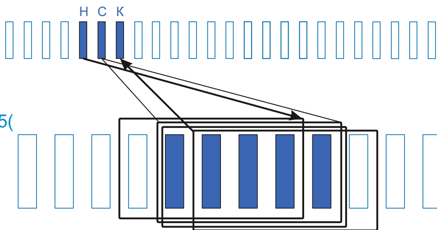
Схема намотки
