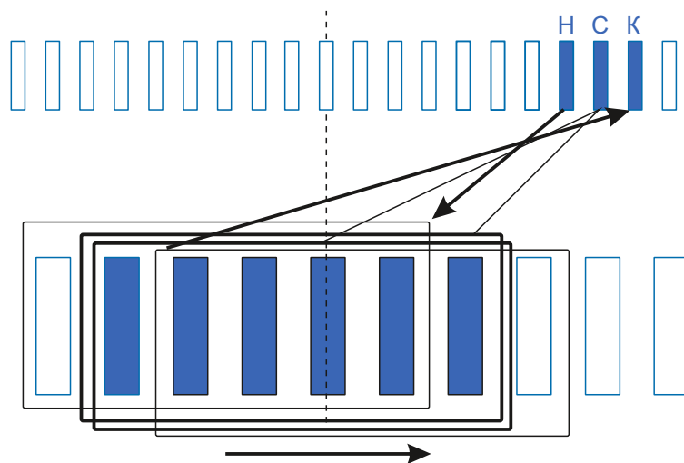
Схема намотки
