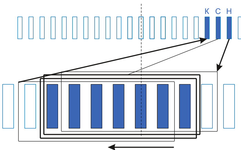
Схема намотки
