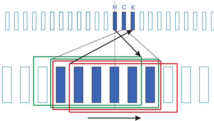
Схема намотки
