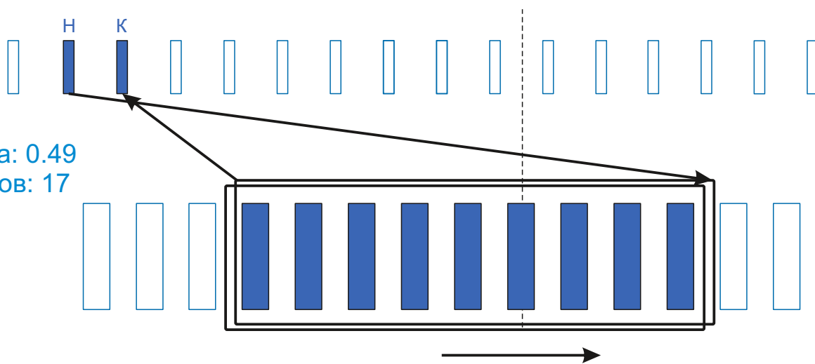
Схема намотки
