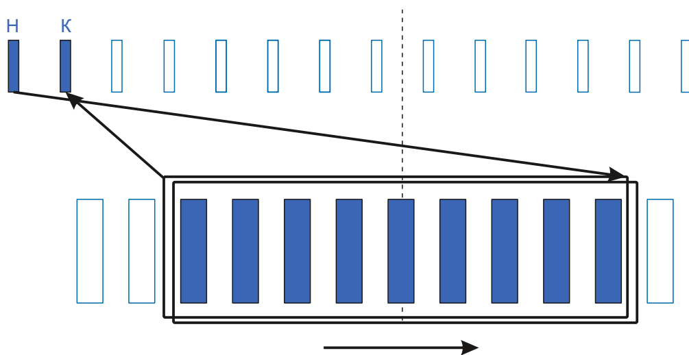
Схема намотки
