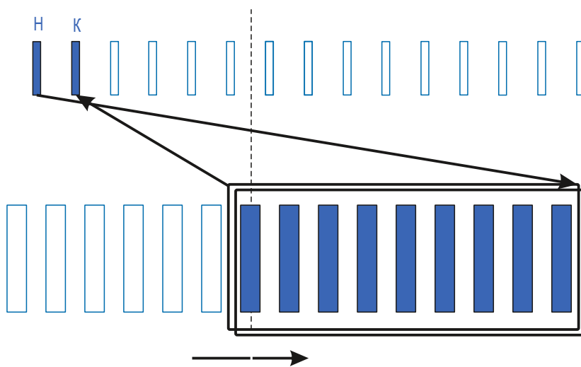
Схема намотки
