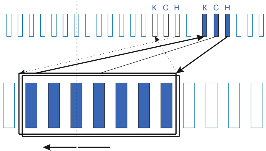
Схема намотки
