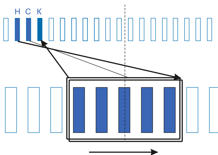
Схема намотки
