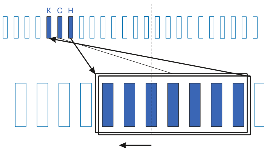
Схема намотки
