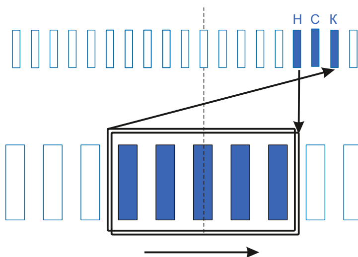
Схема намотки
