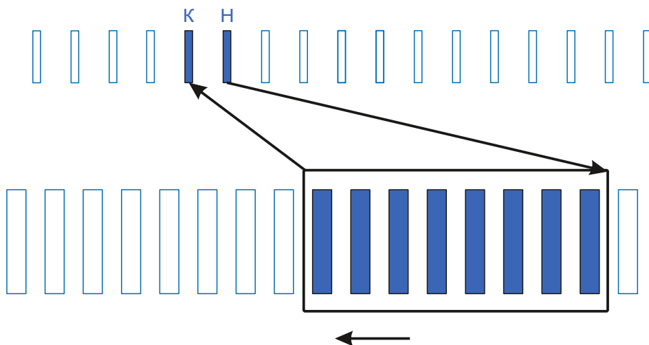
Схема намотки
