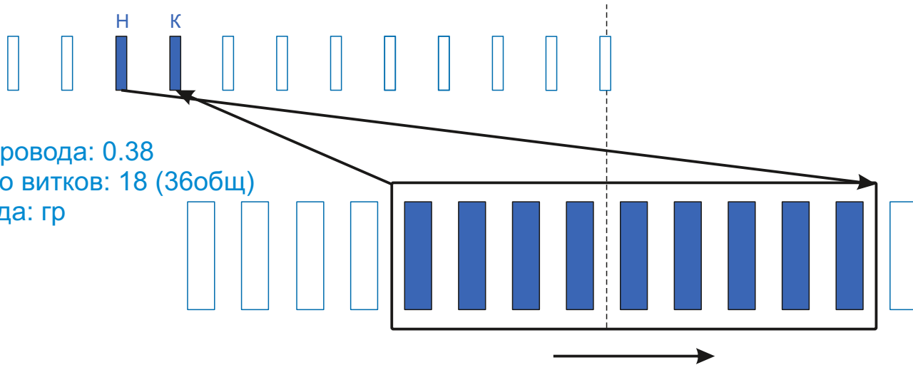
Схема намотки
